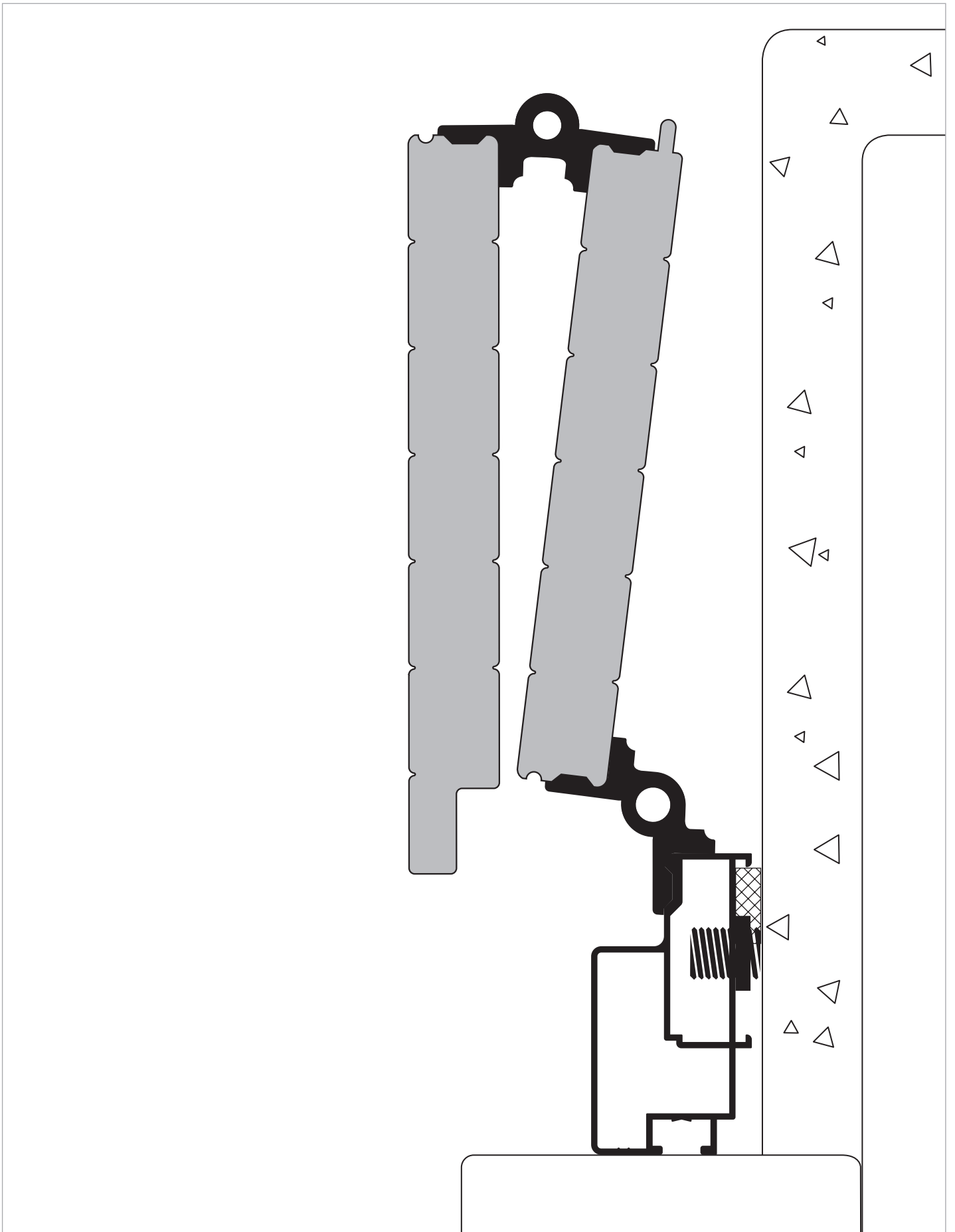
Cassa L 60 a monoblocco con ante da 18 mm a impacchettamento.
