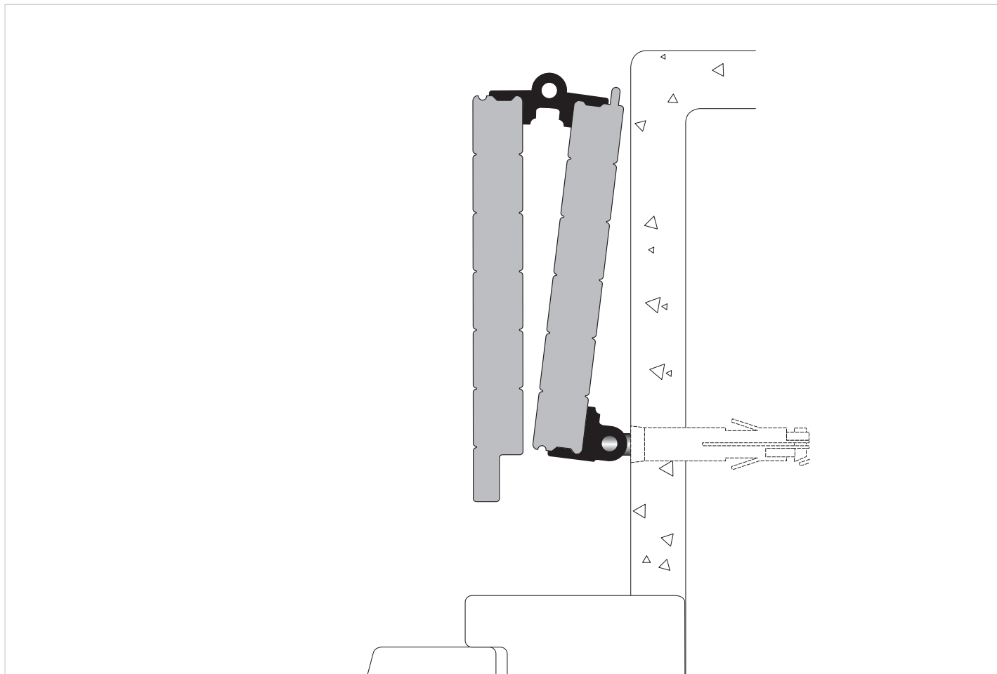
Attacco a muro per ante in luce a impacchettamento - pag. 29
