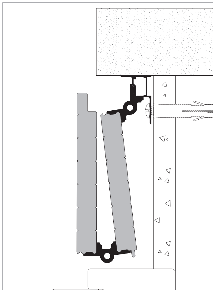
Cassa L 18 per apertura alla vicentina - pag. 27
