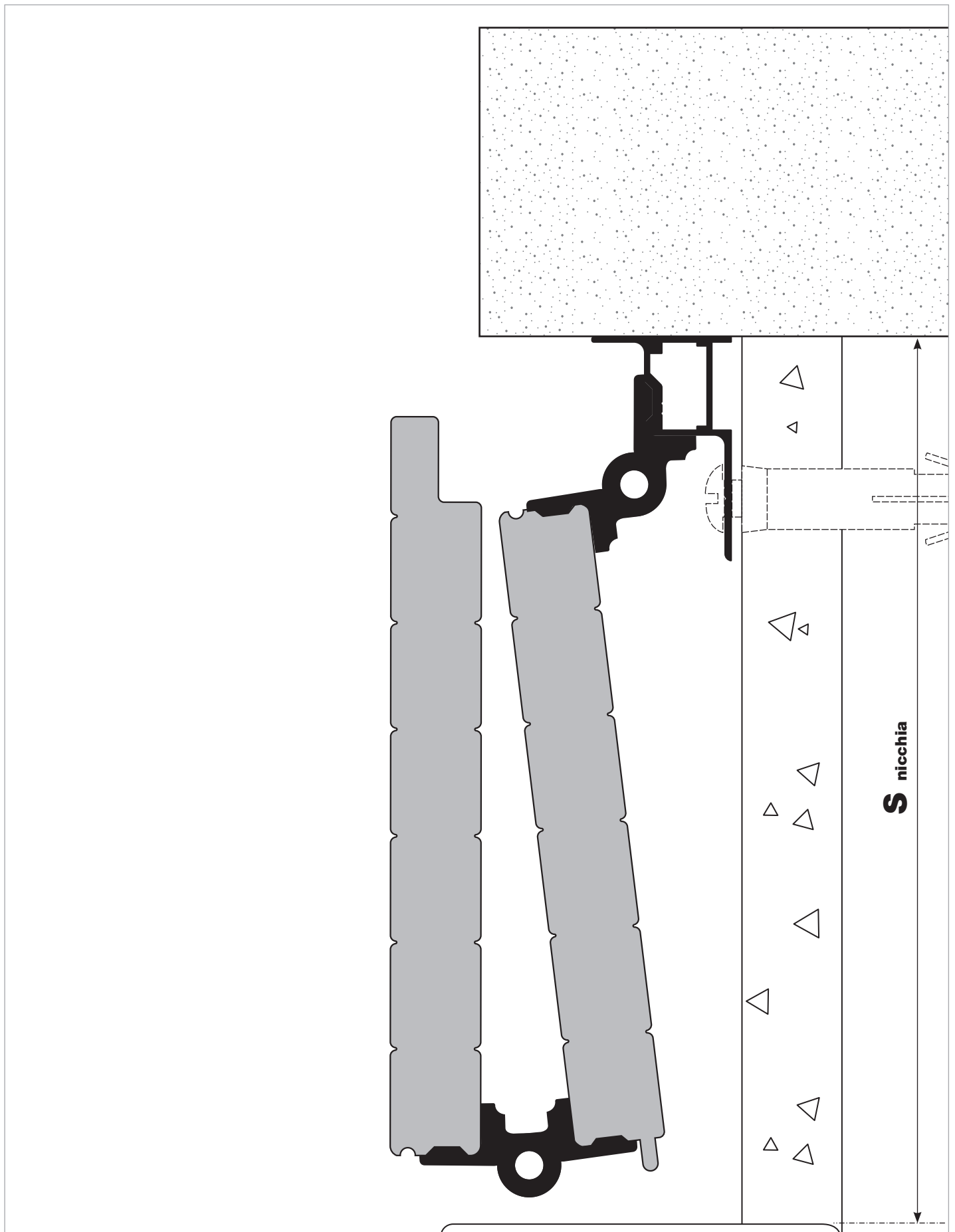
Cassa L 18 per ante in luce da 18 mm in nicchia alla vicentina .
