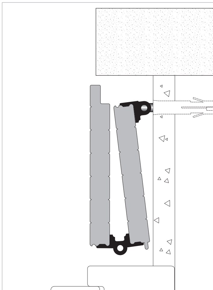
Attacco a muro per apertura alla vicentina - pag. 26
