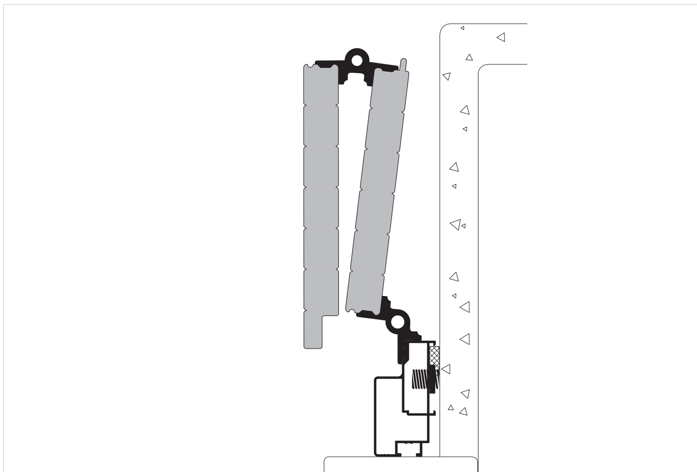
Cassa a L 60 a monoblocco per ante in luce a impacchettamento - pag. 30
