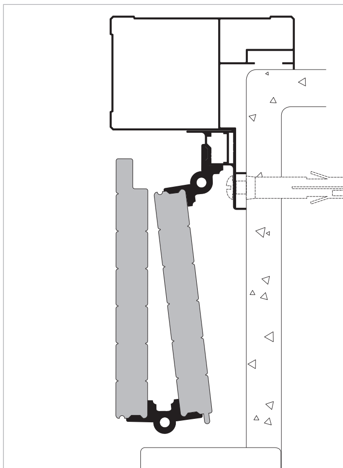
Cassa "Cornise" C 854 per apertura alla vicentina - pag. 28
